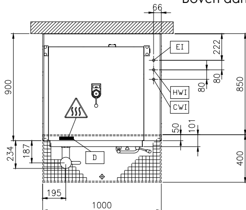
Boven aanzicht
